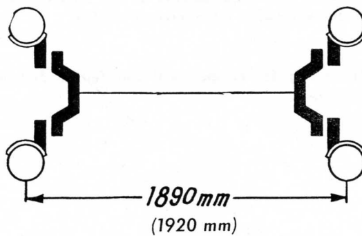
Bild 30 Beispiele für Spurverstellung der Hinterräder Die Klammermaße gelten für 19-30 AS Bereifung Bei Bereifungen ab 11" ist die kleinste Spurweite 1350 mm
